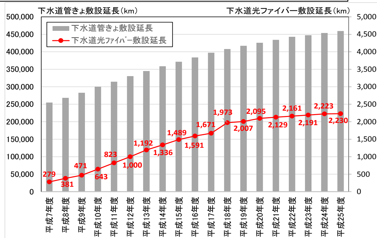
下水道管きょと下水道光ファイバーケーブルの敷設状況
