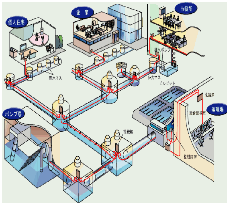
下水道光ファイバーケーブルの敷設イメージ
