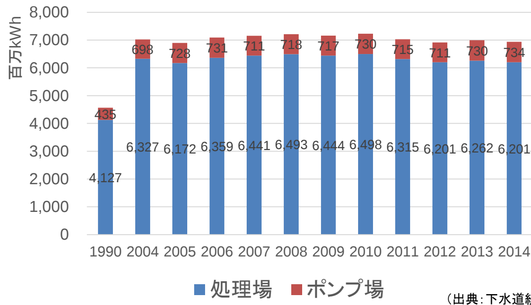
下水道における電力消費量
