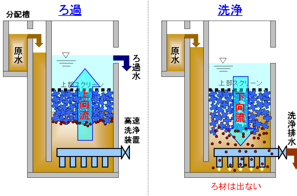
図 3-3 高速ろ過設備概要図②
