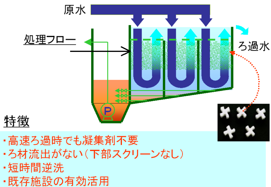
図 3-2 高速ろ過設備概要図①
