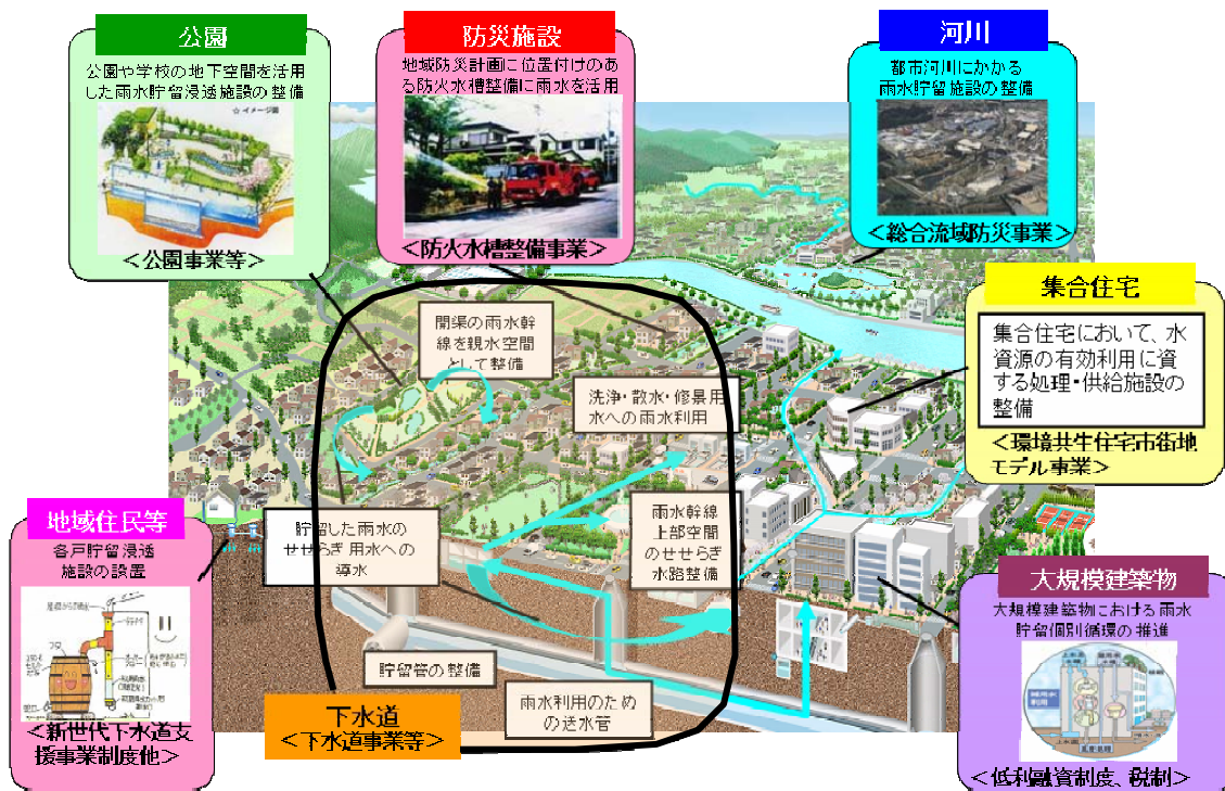
図-20 各事業が連携した雨水利用のための施設整備
