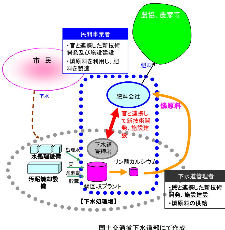
図—2 4 下水道における燐回収システム（イメージ）
