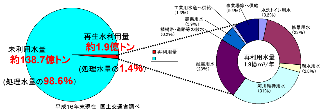
図－22 下水処理水の再利用率とその利用用途
