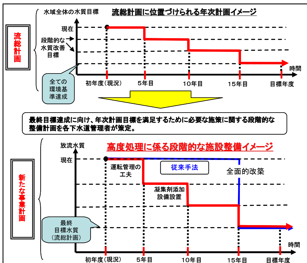
図ー１４ 段階的な水質改善目標と高度処理（イメージ）
