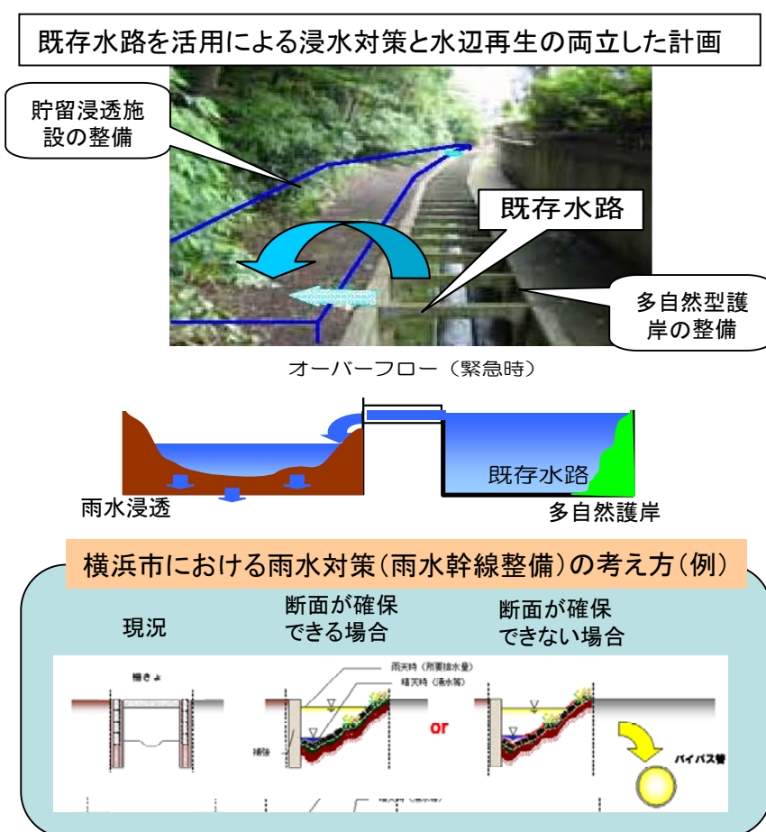
図－１８ 雨水対策における水面の確保（横浜市）
