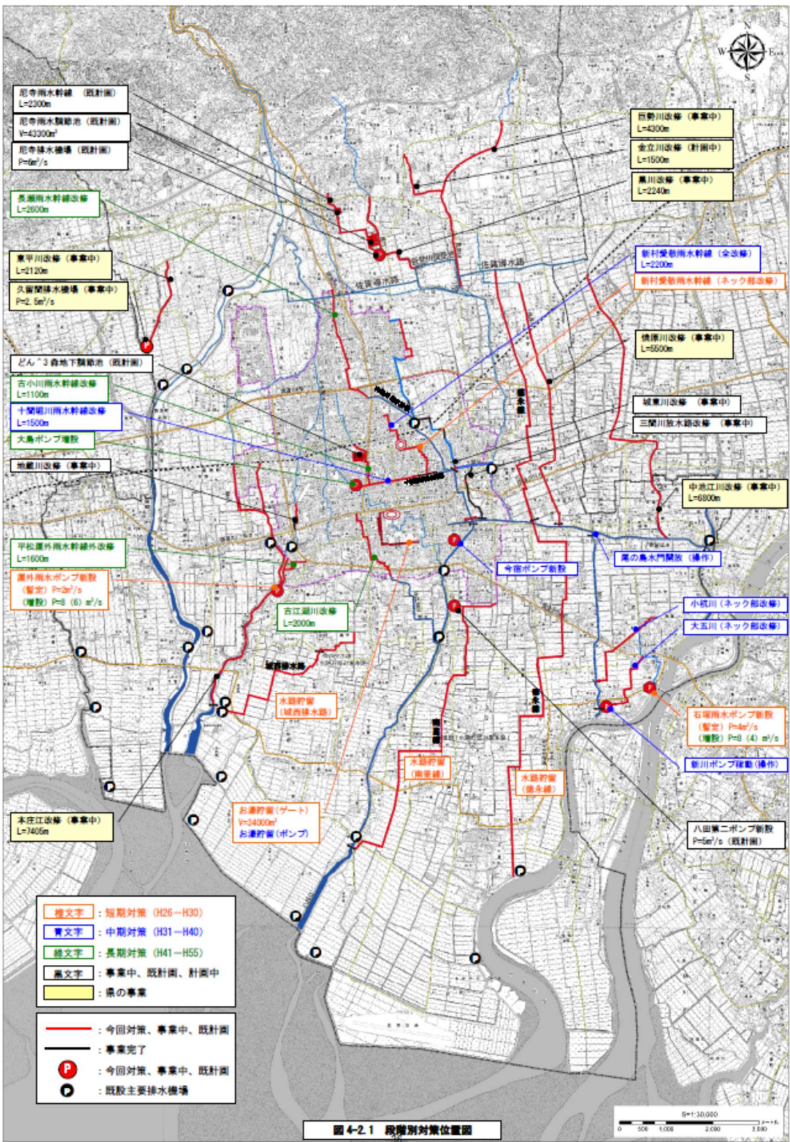
図 2 - 1 0 雨水管理総合計画マップの例（佐賀市）
