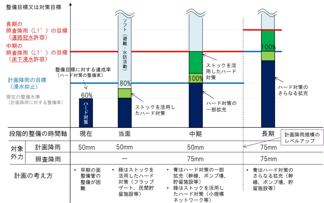
図2-5 整備目標、対策目標の達成に向けた段階的対策計画の例
