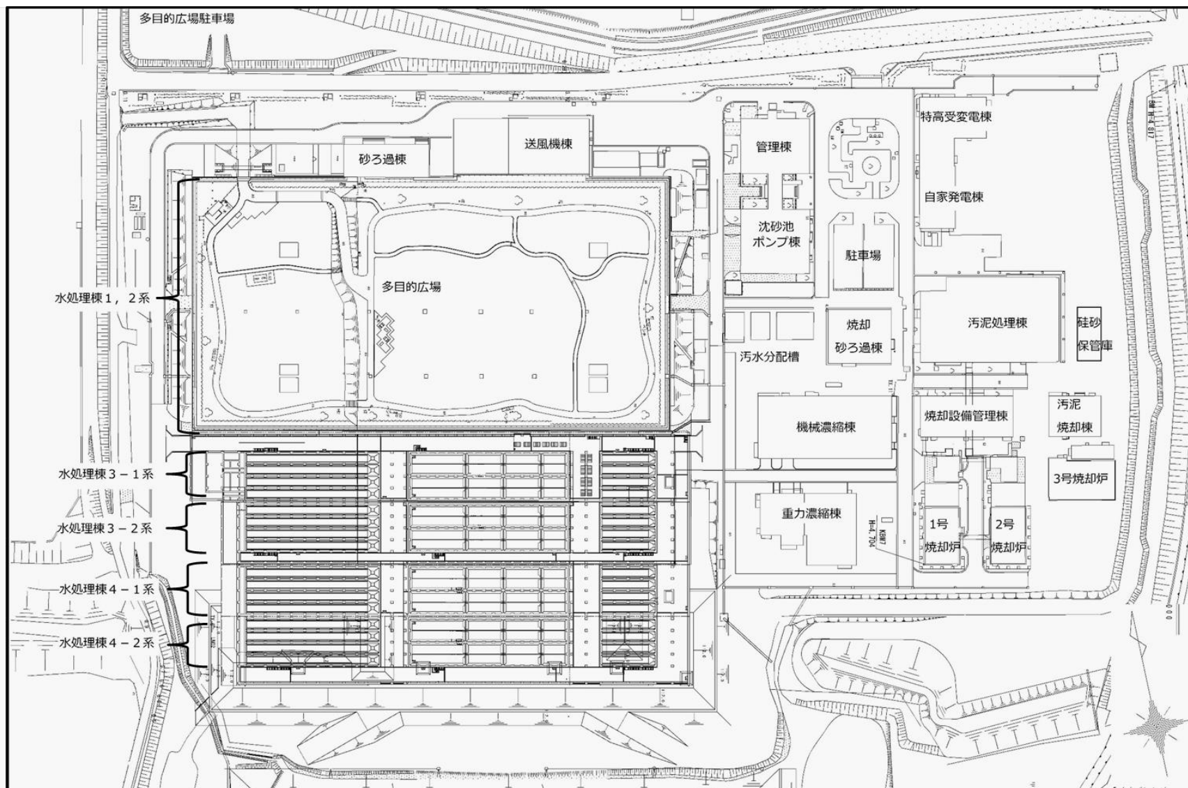
別紙 4-2 西遠浄化センター一般平面図（拡大）
