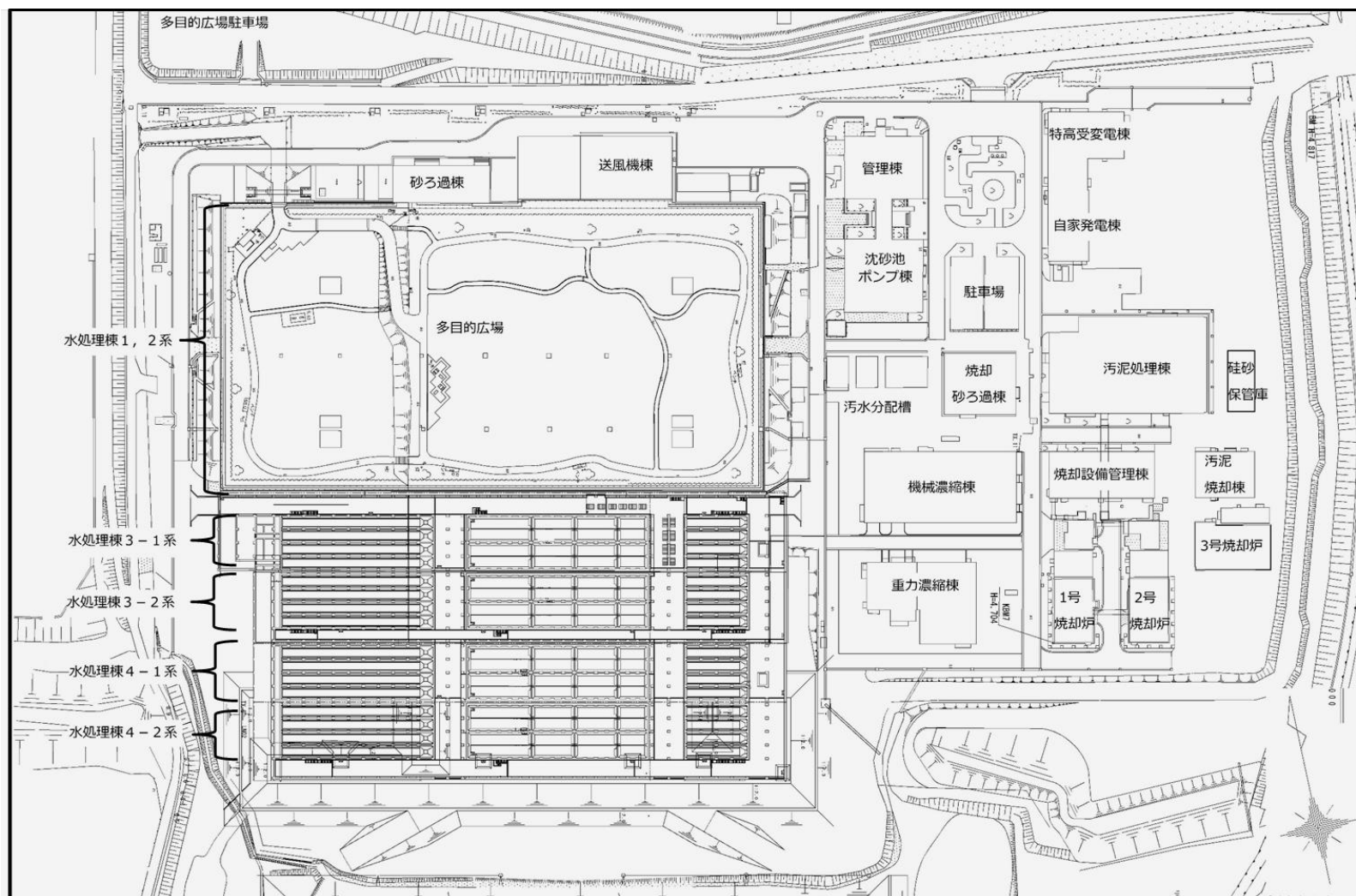
別紙 1－2 西遠浄化センター一般平面図（拡大）
